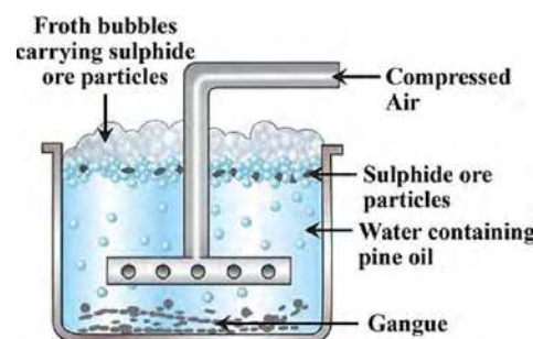
Fig: Froth floatation
