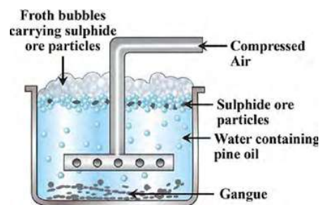
Fig: Froth floatation
