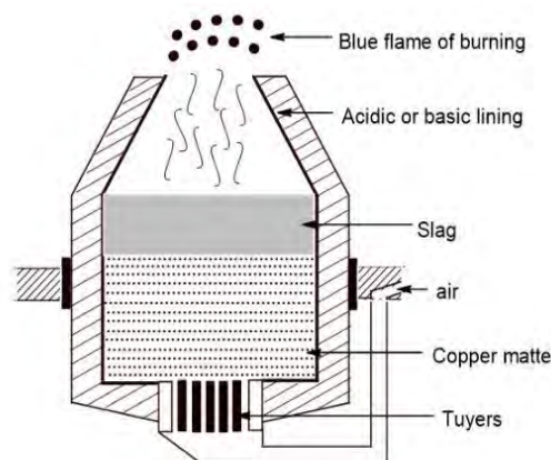
Fig: Bessemer converter
