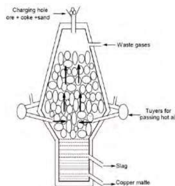
Fig: Blast Furnace
