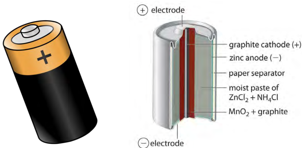
Fig 5.7.1: Leclanche dry cell
