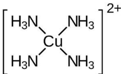
Tetraamminecopper (II) ion
